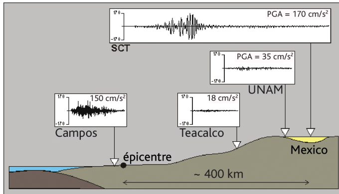
Figure 8.1. Exemple d'effets de site dans la zone lacustre de Mexico (PGA : Peak Ground Acceleration). © Jean-François Semblat.
